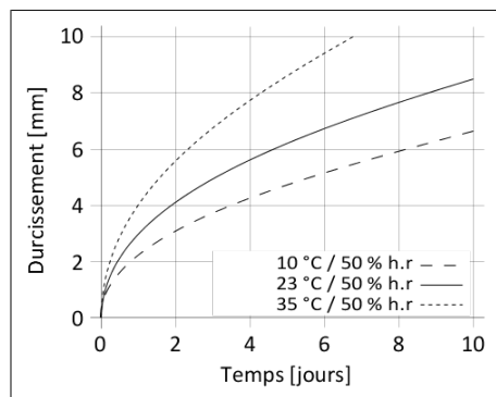
Diagramme 1: Vitesse de polymérisation du Sikaflex®-554
