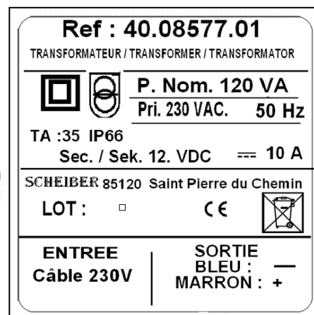
Plaque signalétique
